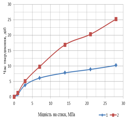
Рис. 5. Кінетика набору міцності каменю на основі романцементу з добавкою: 1 – 2 % лимонної кислоти; 2 – 1 % соди та 1 % борної кислоти
