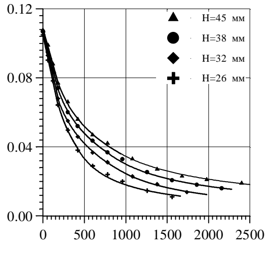
Рис. 3. Кінетика фільтраційного сушіння амофосу ( t = 50^{\circ}C ; v_0 = 1,26 м/с)
