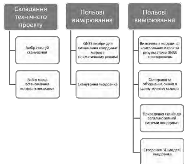
Рис. 3. Технологічна схема наземного лазерного сканування острівних льодовиків
