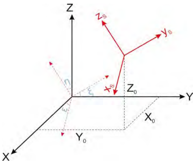
Рис. 6. Схема перетворення координат
