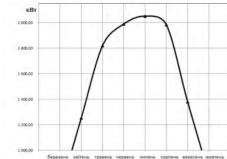
Рис. 2. Надходження теплоти від сонячного випромінювання в побутовий біореактор протягом ТПР
