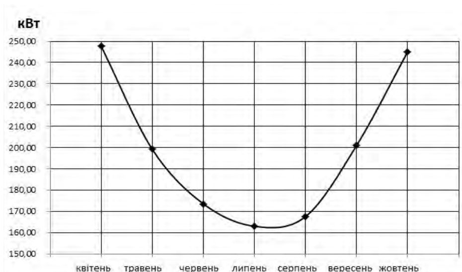
Рис. 3. Кількості теплоти для підігріву біореактора в ТПР
