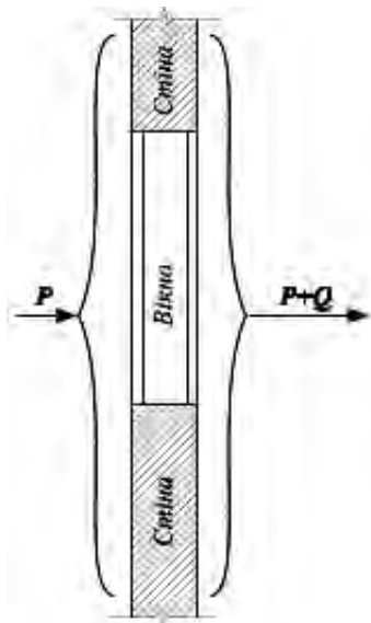
Рис. 1. Схема теплових потоків через огороження будівлі
