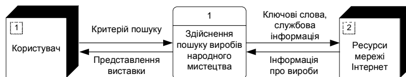
Рис. 2. Контекстна діаграма потоків даних
