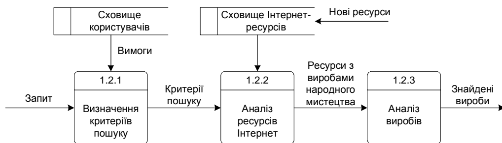
Рис. 4. Декомпозиція діаграми потоків даних другого рівня процесу “Здійснення пошуку виробів”
