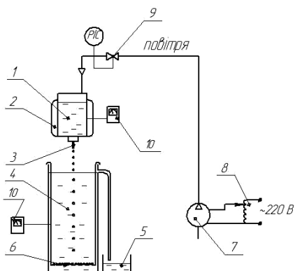
Рис. 1 Принципова схема лабораторної установки: 1 – реактор; 2 – термостат; 3- циліндрична насадка; 4 – збірник мікрогранул; 5 – збірник масла; 6 – перфорована перегородка; 7 – компресор; 8- електротрансформатор; 9 – стабілізатор тиску; 10-термометр
