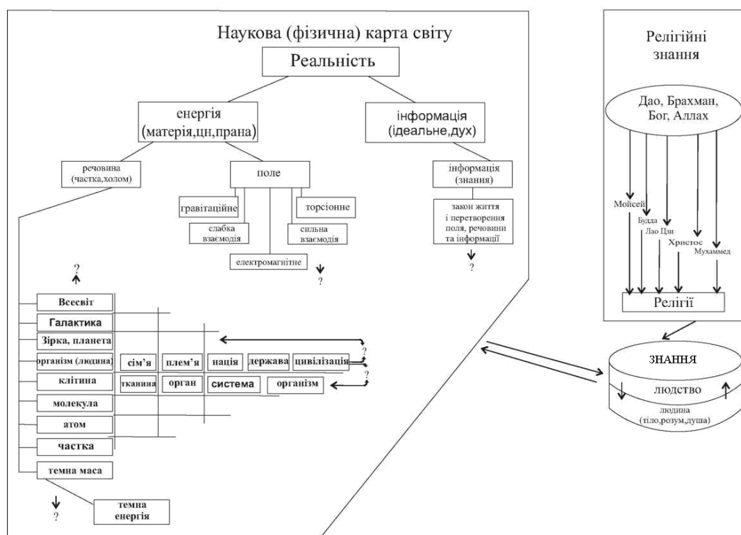
Рис.1 Структура елементів Реальності
