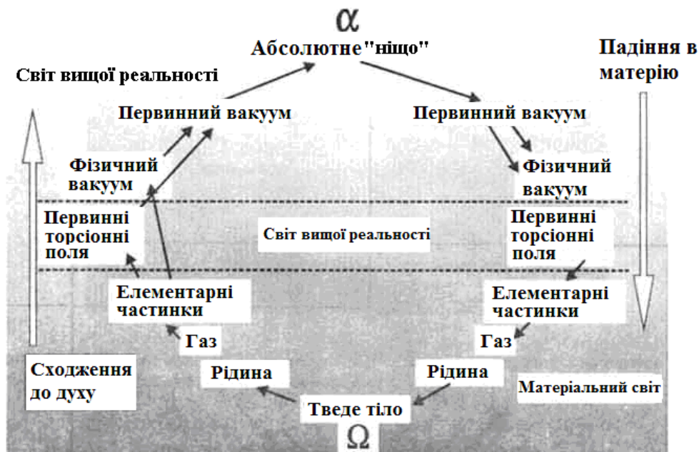
Рис.4. Коло Сансари в теорії фізичного вакууму.
