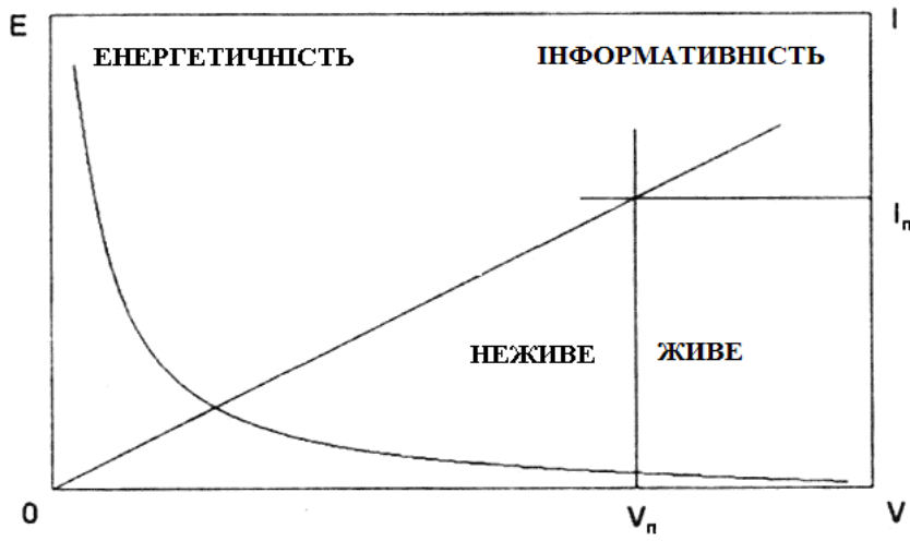
Рис.2. До поняття вітальності систем
