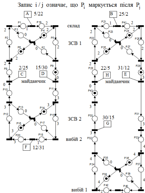
Рис.1. Граф синхронізації системи склад-вибій
