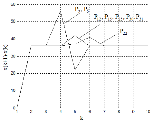
Рис.2. Компенсація збурення в системі
