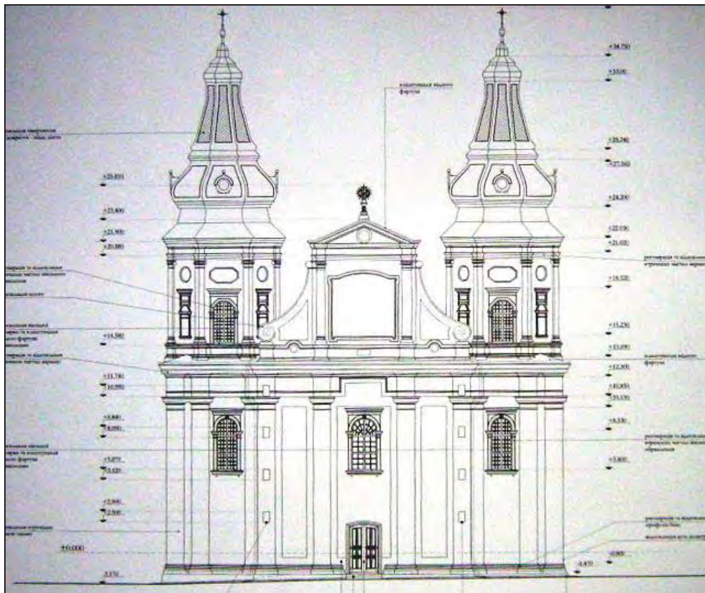
Рис. 10. Ескізний проект реставрації пам'ятки архітектури XVII ст. Успенського костелу в м. Угневі. Науково-проектна робота НДЛ-104 у 2008 р. Автори: Ю. Дубик, О. Рибчинський, І. Бокало та ін.
