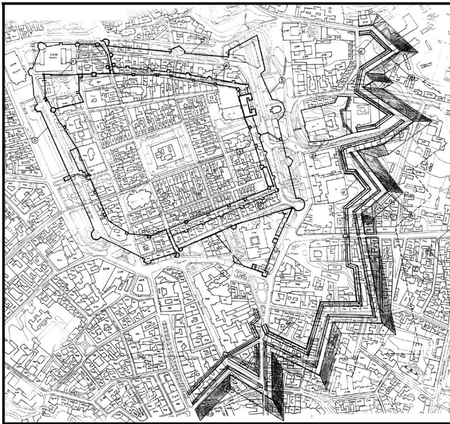
Рис. 6. Науково-прикладні розробки кафедри: реконструкція оборонної лінії Яна Беренса, створеної для укріплення львівського середмістя наприкінці XVII ст. (оборонний бастионний пояс зіствлено із сучасною топографічною підосною). М. Бевз, асп. І. Оконченко
