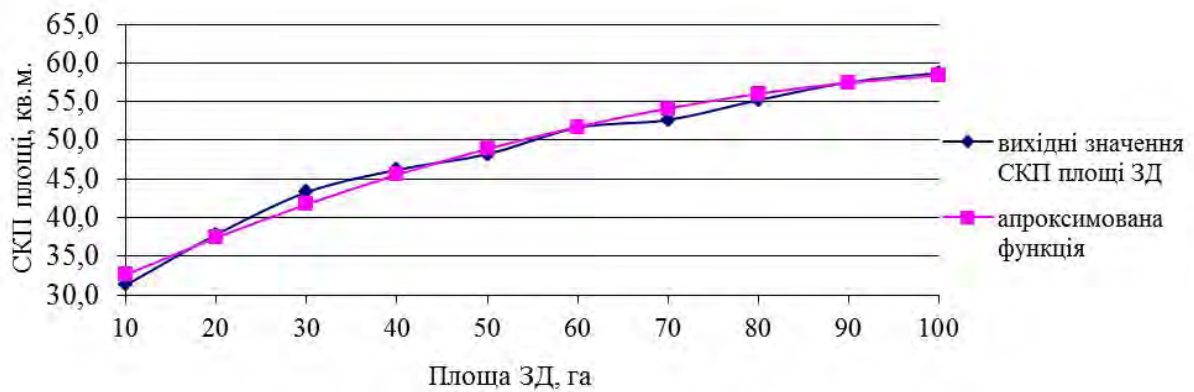
Рис. 4. Графік апроксимованої квадратичної функції при k = 3 для площ ЗД 10–100 га
