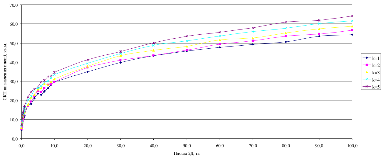
Рис. 1. Графіки залежності середніх квадратичних похибок площ земельних ділянок від значення їх площі і коефіцієнта видовженості k (за даними [12])
