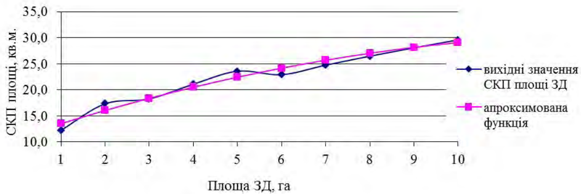
Рис. 3. Графік апроксимованої квадратичної функції при k = 1 для площ 3Д 1-10 га
