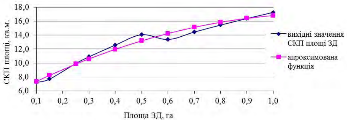
Рис. 2. Графік апроксимованої квадратичної функції при k = 5 для площі ЗД 0,1-1 га
