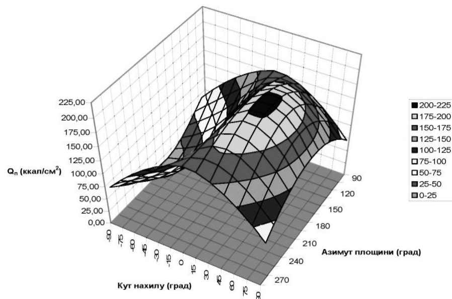
Рис. 1. Залежність надходження СР від азимута і кута нахилу за рік ( Q_n=f(A, \omega) )
