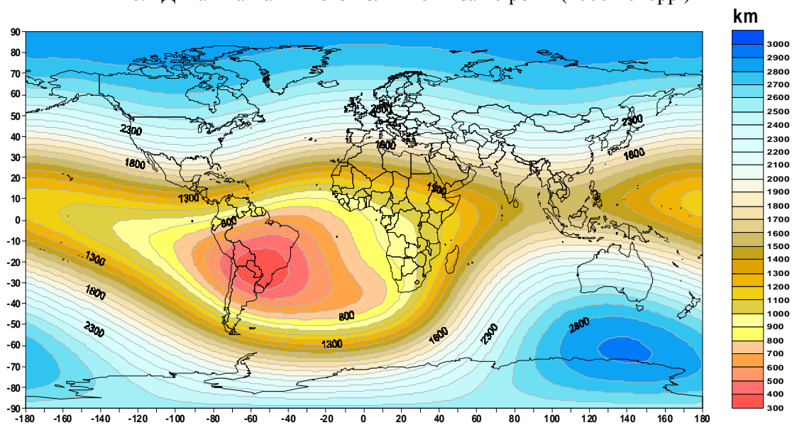
Рис.5 Еквіпотенційна поверхня з індукцією поля B=20000 нТл.
