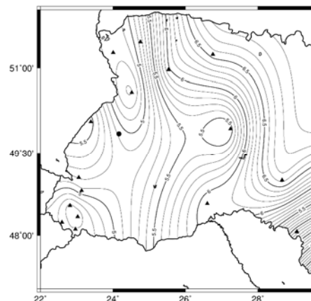
Рис. 1. Магнітне схилення D приведене на епоху 2010 року (•- обсерваторія "Львів")
