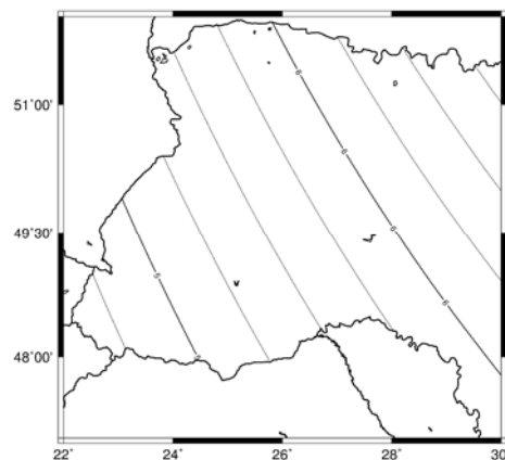
Рис. 2. Магнітне схилення D по моделі IGRF 2011 на епоху 2010 року
