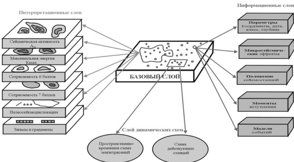
Рис.1. Блок-схема структуры ГИС “Сейсмичность Магаданской области”
