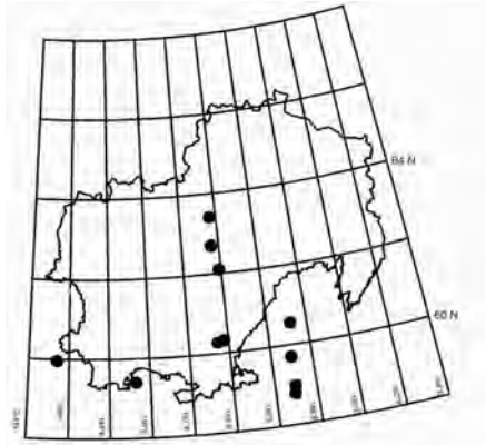
Рис.2. Распределение эпицентров землетрясений за период 1988-1997 гг., ● - K \geq 12,0
