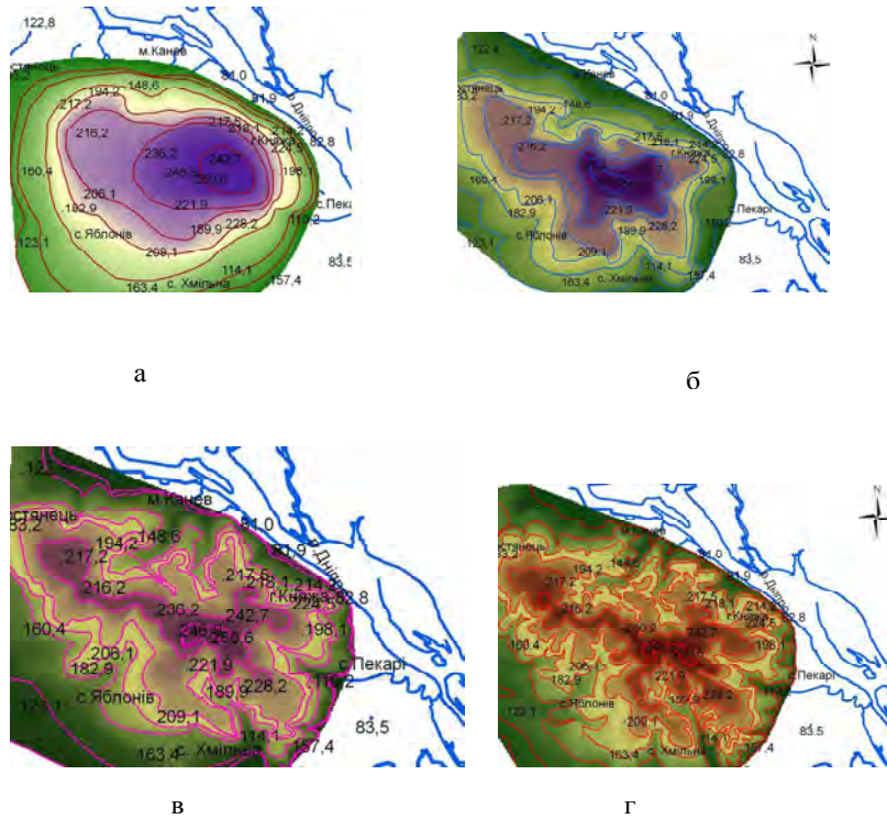
Рис. 1. Базисні поверхні рельєфу Канівського Придніпров'я: а – п'ятого порядку, б – четвертого порядку, в – третього порядку, г – другого порядку.
