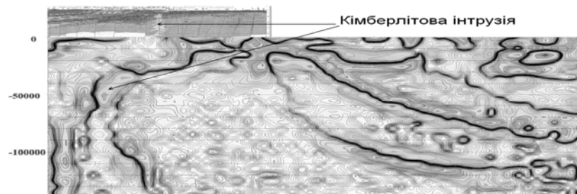
Рис. 2. Томографічний розріз за параметром “густина-намагніченість” по регіональному профілю РП-5 (фрагмент), автор С.Г. Слоницька
