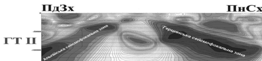
Рис. 1. Томографічний розріз за параметром “густина-намагніченість” по геотраверсу II (фрагмент), автор С.Г. Слоницька
