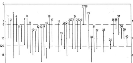
Рис. 1. Розподіл хвилеводів в земній корі Українського (1-17), Балтійського (18-32), Індійського (33), Канадського (34-40) щитів. \Delta V_p = 0,1-0,7 км/с (0,1-0,22 км/с), \Delta H = 3-15 км, H_{\text{мін}} = 5-12 км [Трипольский, Шаров, 2004].
