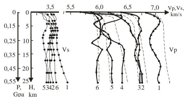
Рис. 2. Зміна V_{p,s} = f(P,T) = f(H) з глибиною для різних гранітоїдів:
