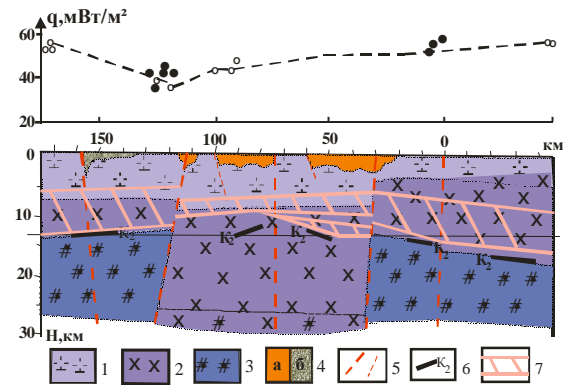
Рис. 3. Фрагмент схематичного розрізу речового складу земної кори ділянки геотраверса ІV:
