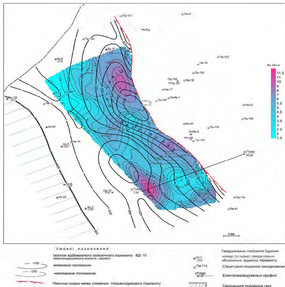
Рис. 2. Карта поздовжнього опору та структурна карта горизонту VD-10
