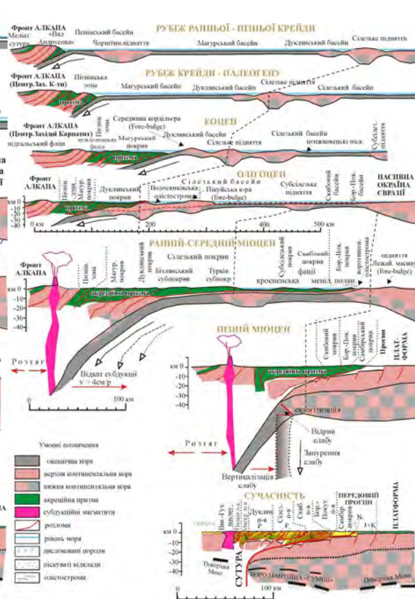
Рис. 2. Палінспастичні розрізи західного сегменту Українських Карпат. Склав О. М. Гнилко з використанням матеріалів [Астахов, 1989; Тектоно-магматическая..., 1995; Csontos, Voros, 2004; Oszczyzko, 2006; і ін.]
