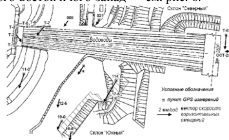
Рис. 6. Вектора скоростей горизонтальных смещений центральной части гидротехнического сооружения ЗАГАЭС
