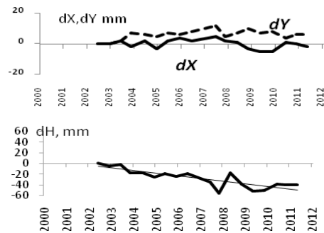
Рис. 3. Графики временного хода компонент ( dX – север-юг, dY – восток-запад, dH – поднятие-опускание) пункта Т-2 за 2002-2011 гг
