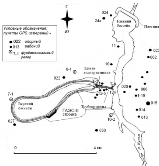
Рис. 1. Схема расположения пунктов ГНСС измерений на территории ЗАГАЭС-1
