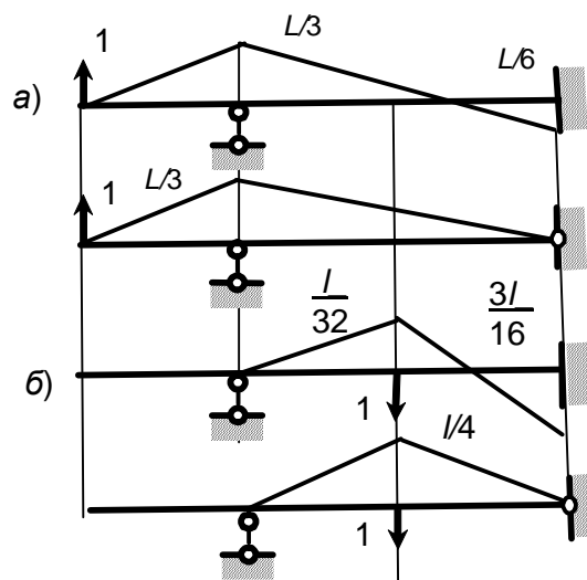
Рис. 4. Единичные эпюры вычисления перемещений по правилу Верещагина
