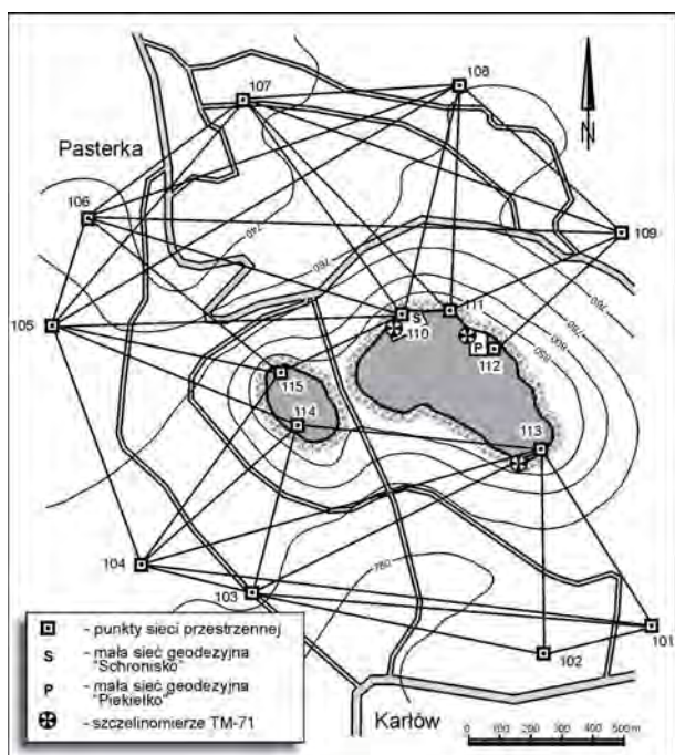
Rys. 1. Szkic sieci pomiarowej "Szczeliniec" (Mąkowski i inni, 2005, na podstawie wcześniejszych opracowań)
